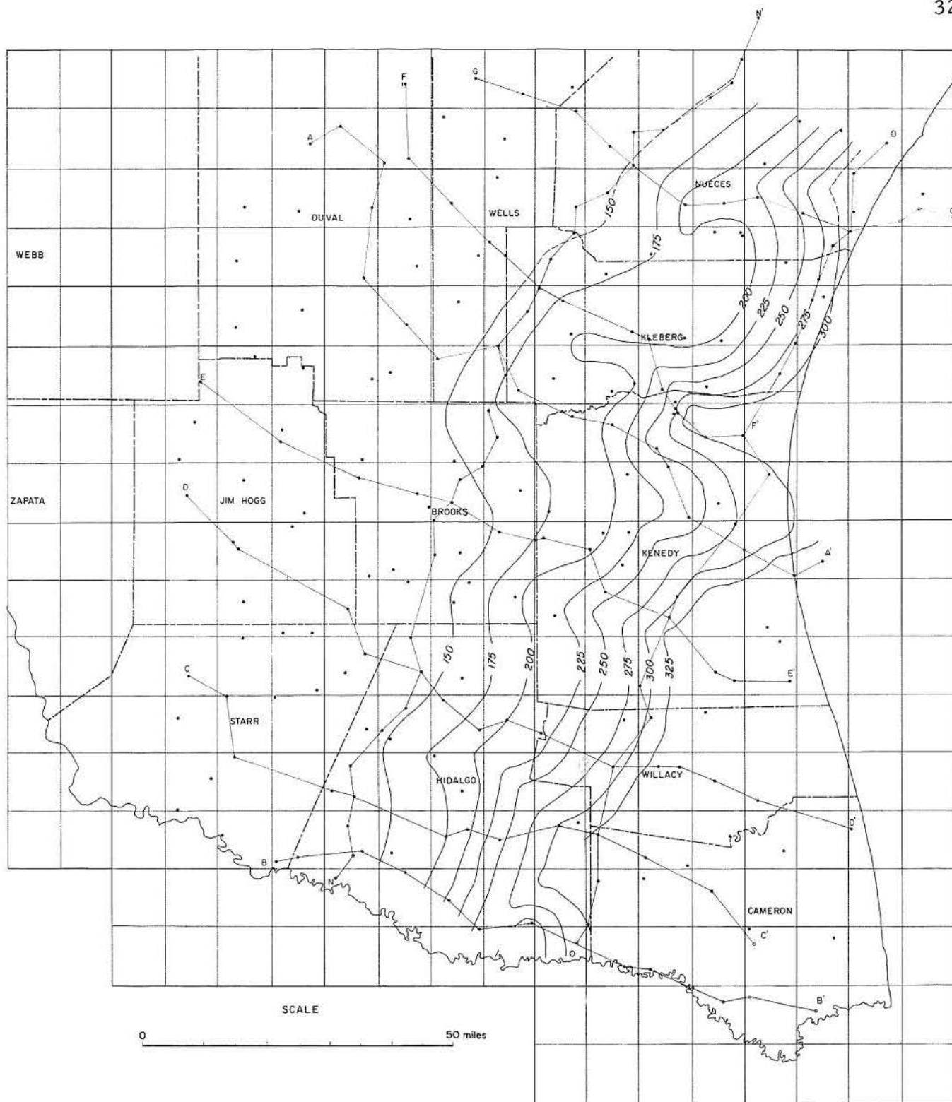
Fig. 24. Isothermal map on T5 datum.
