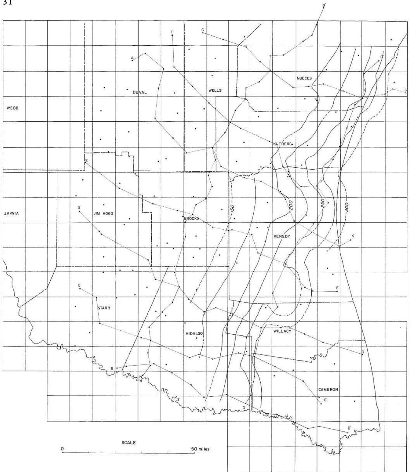
Fig. 23. Isothermal map on T4 datum.
