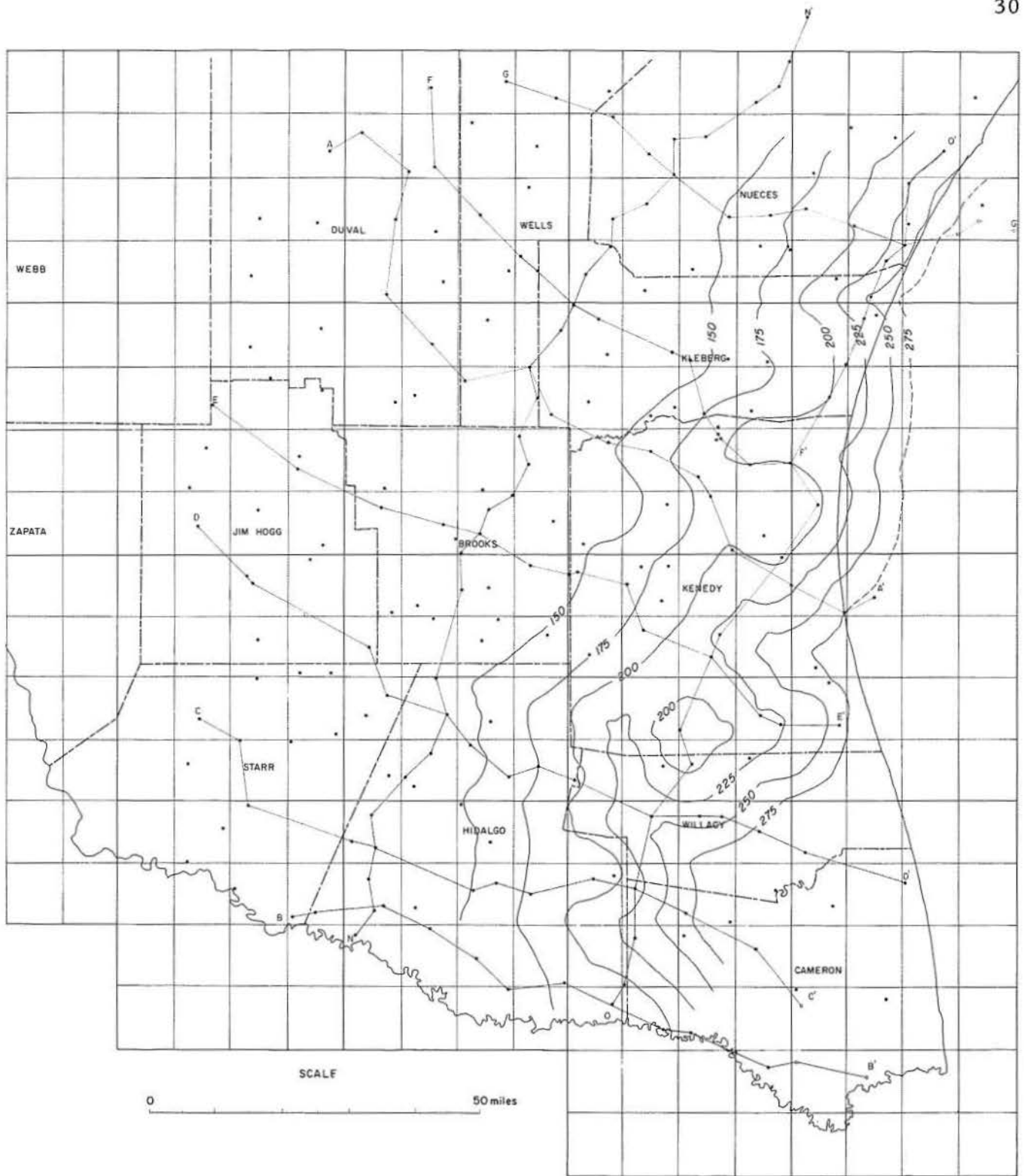
Fig. 22. Isothermal map on T3 datum.
